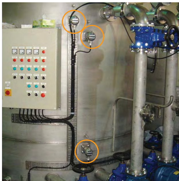
Interruptores de nível Tipo: A 01 051E15
