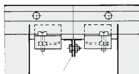
PORMENOR DE LIGAÇÃO ENTRE TROÇOS
